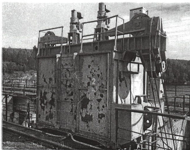
Рис. 1. Корпус лебедки
